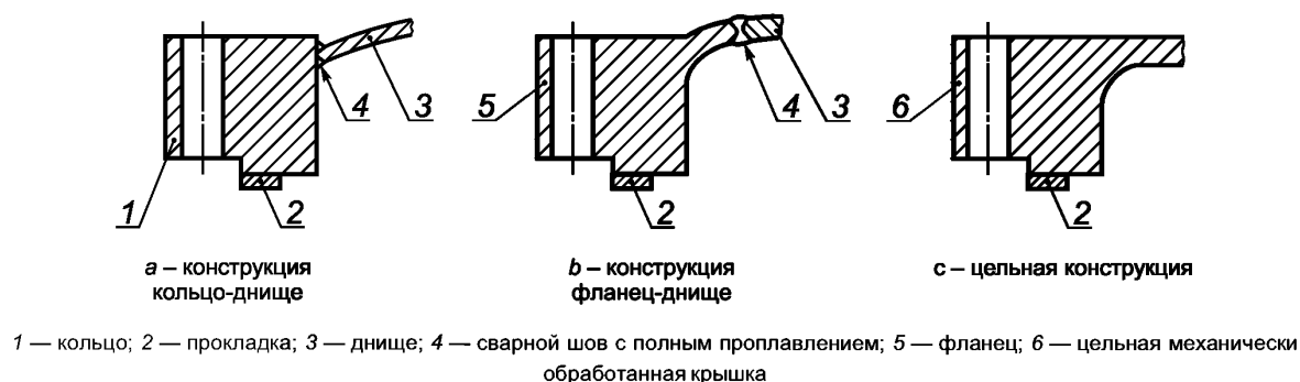
Рисунок 4 — Типовые конструкции крышек плавающих головок
